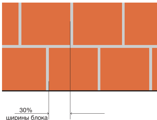
Рис. 9. Минимальная перевязка вертикальных швов
